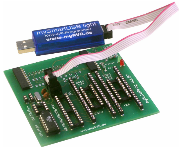
Abbildung / picture: myMultiProg MK2 mit mySmartUSB light über ISP myMultiProg MK2 with mySmartUSB light via ISP
