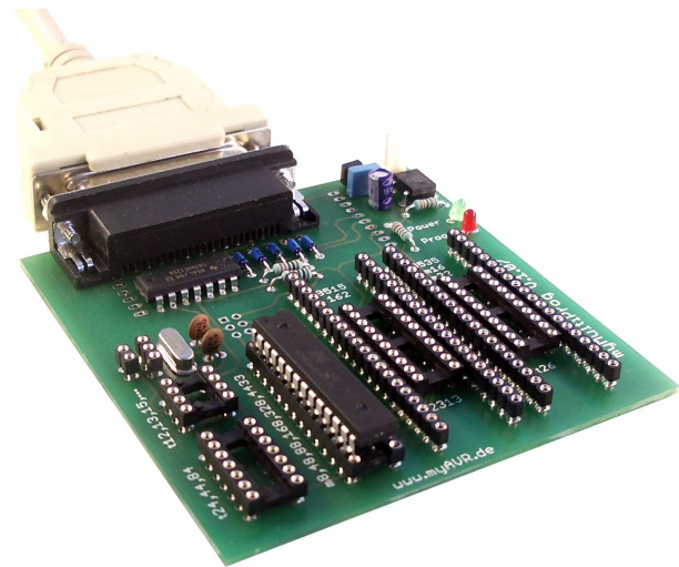
Abbildung / picture: myMultiProg MK1 mit ATmega8 myMultiProg MK1 with ATmega8
