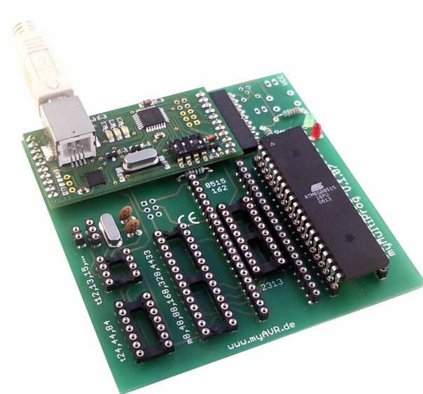
Abbildung / picture: myMultiProg MK2 mit ATmega8515 myMultiProg MK2 with ATmega8515
