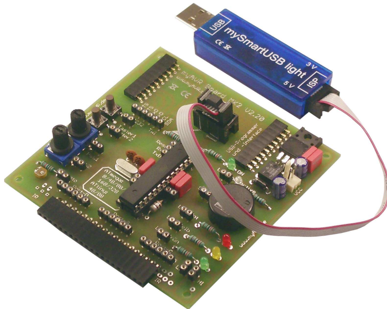
Abbildung / picture: myAVR Board MK2 mit mySmartUSB light myAVR board MK2 with mySmartUSB light
